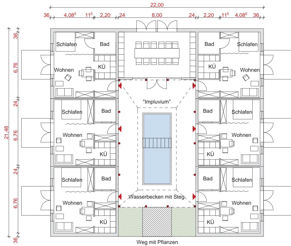
GRUNDRISS KLEINWOHNUNGEN M 1:200
