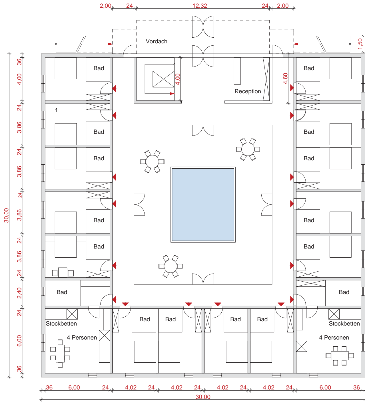
GRUNDRISS HERBERGE / HOSTEL M 1:200
